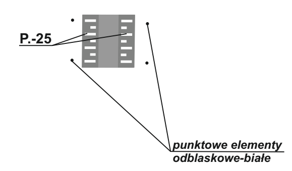
Wzór oznakowania progu
