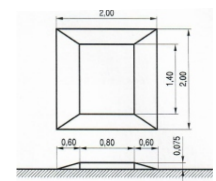
Przekrój progu U-16 wyspowego
