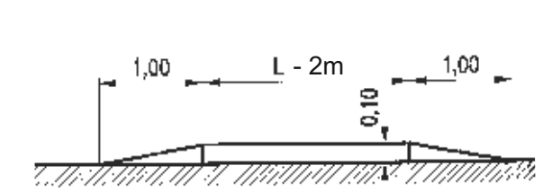
Przekrój progu U-16c
